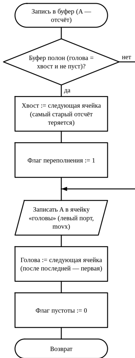
Рис. 3.5. Схема алгоритма: Запись отсчёта в кольцевой буфер
