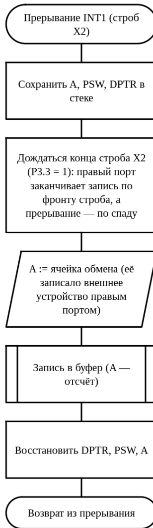
Рис. 3.6. Схема алгоритма: Обработчик прерывания INT1: приём отсчёта X2 от внешнего устройства
